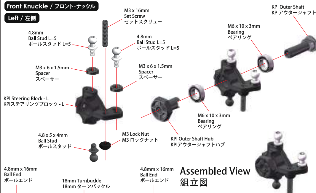
4.8 x 5 x 4mm Ball Stud (2) 4.8 x 5 x 4mm ボールスタッド (2)
