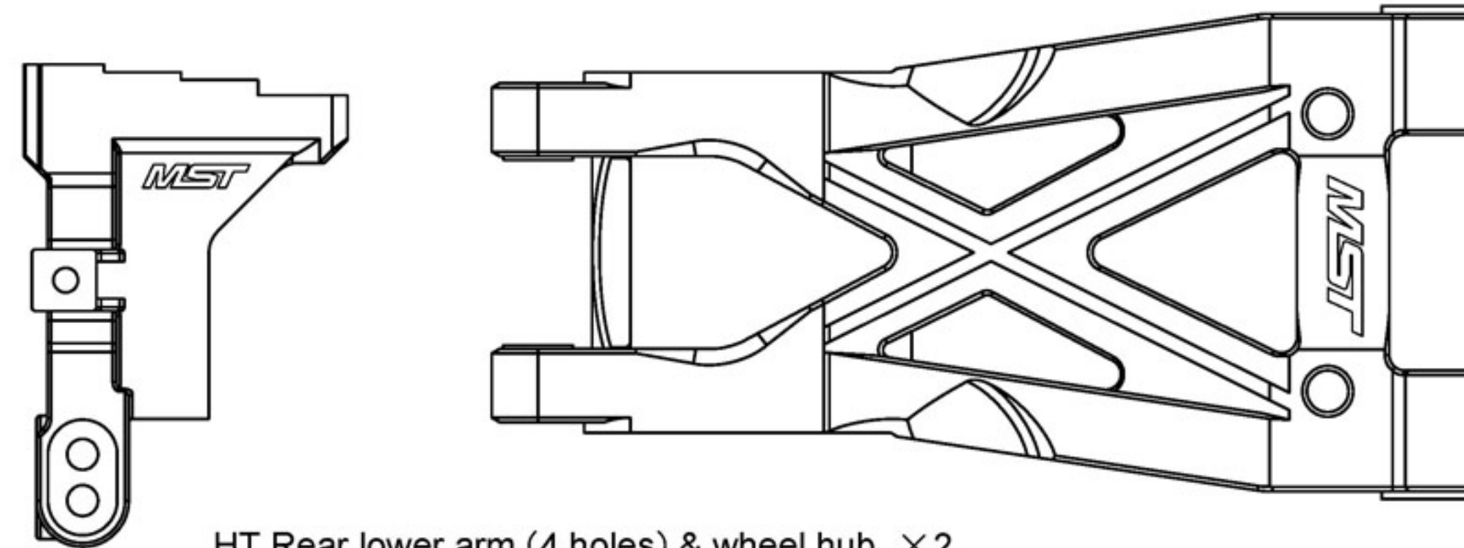
HT Rear lower arm (4 holes) & wheel hub ×2 HT 後下擺臂 (4孔) & 輪座 210070
