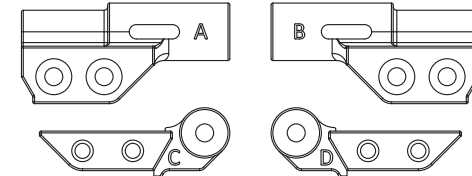
HT Upper arm HT 上擺臂 210058
