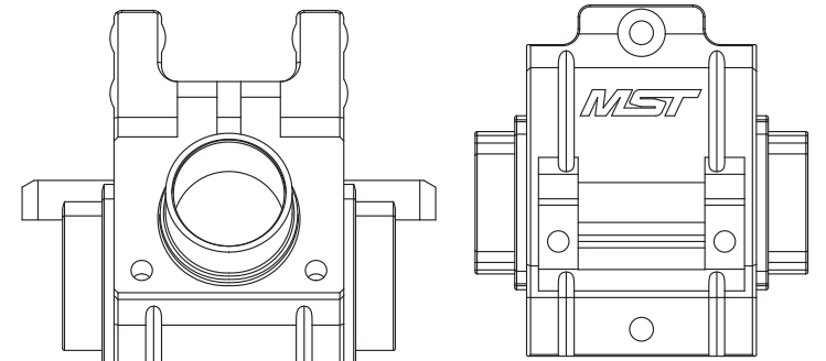
FXX Rear gear box set FXX 後齒箱組 210077
