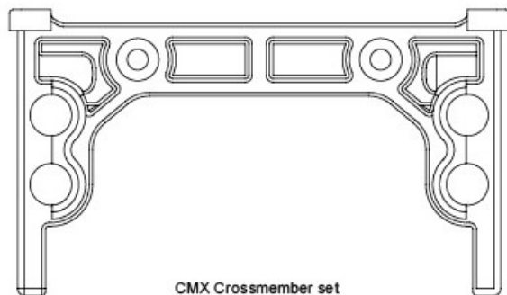
CMX Crossmember set CMX 橫樑組 230019
